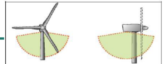
Abbildung 1: batsorder 2.0 inkl. WKA-Erweiterung 1.0 in der Bodenwanne einer Enercon E62
