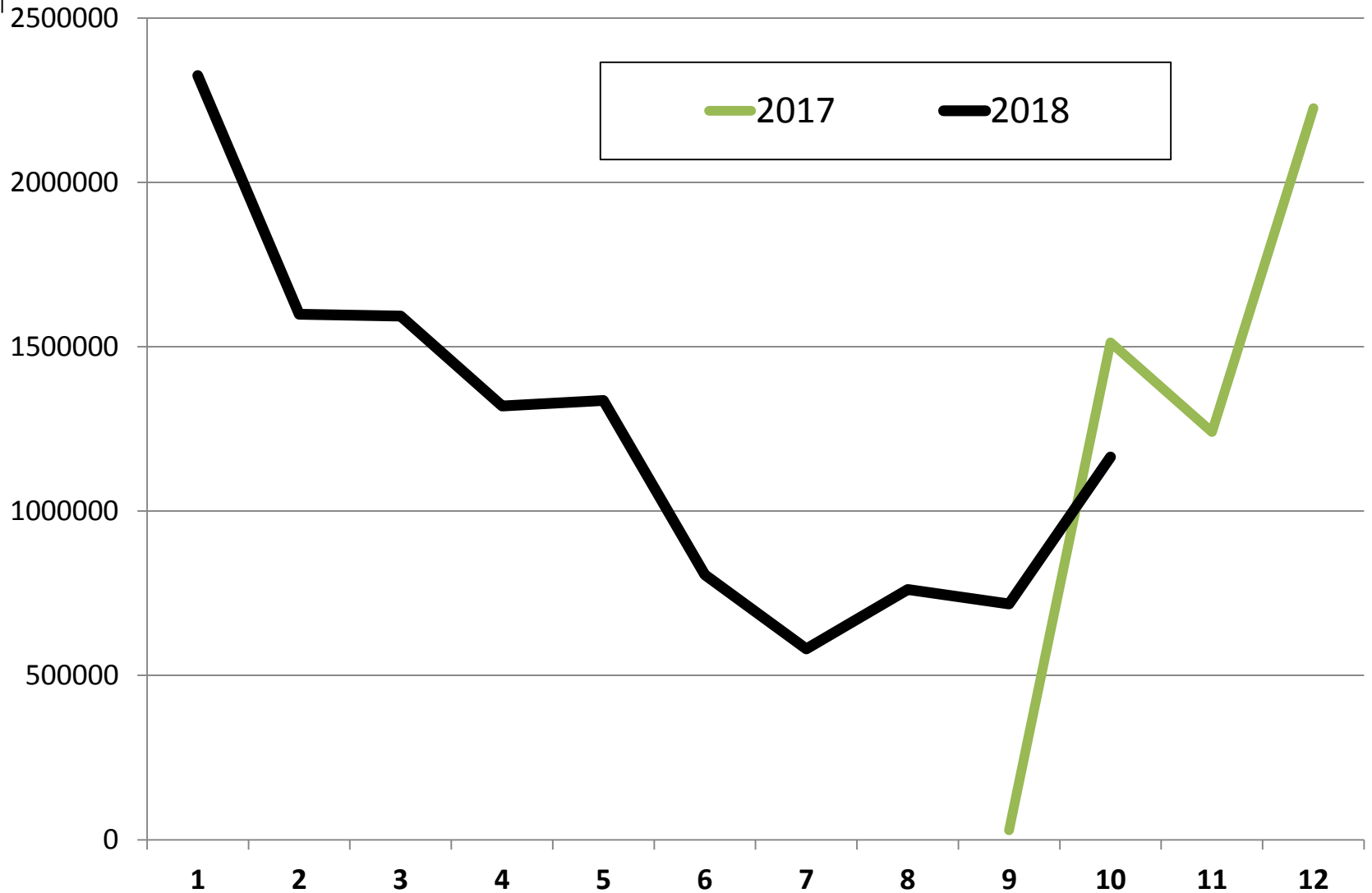
Monatlicher Ist-Ertrag Windpark Binsfeld
